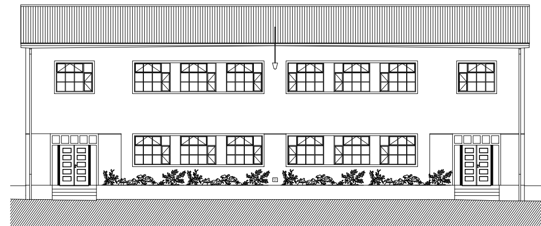
Alçado Sul
