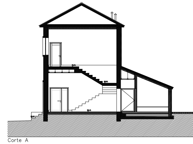
Corte A
